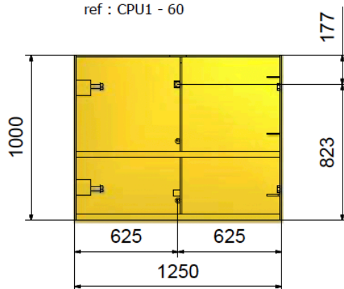
Panneau 1,25 x 1,00 ht ref : CPU1 - 60
