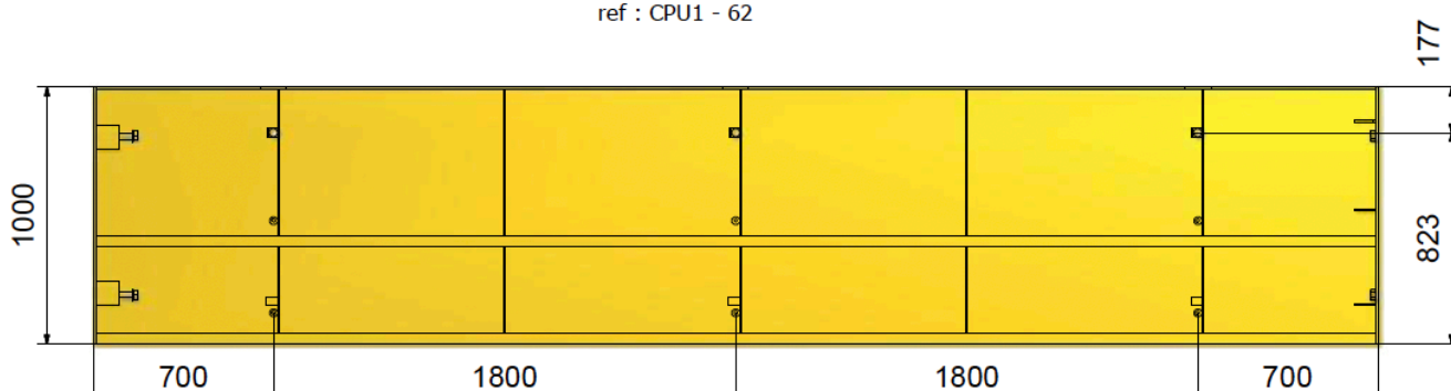
Panneau 5,00 x 1,00 ht ref : CPU1 - 62
